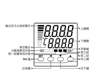
圖3. 面版說明
