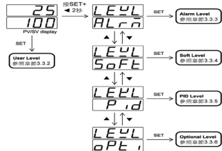
圖5. 參數流程
