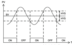
圖11. ON/OFF 控制動作
