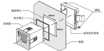
圖1. 盤面安裝
