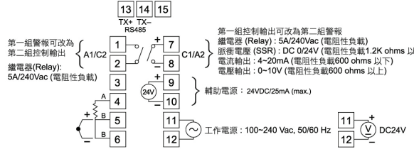
圖2. 配線圖
