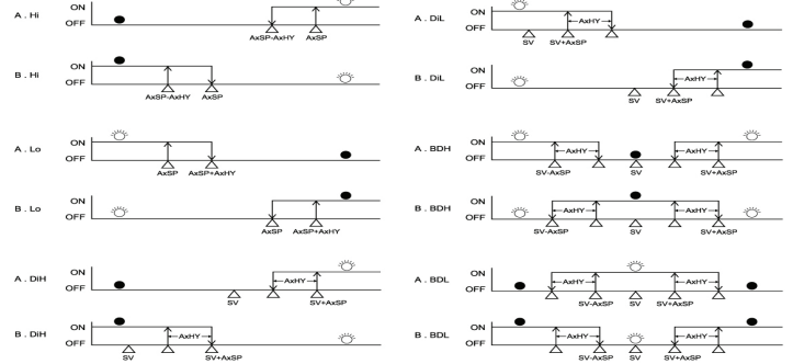
圖7. 警報方式
